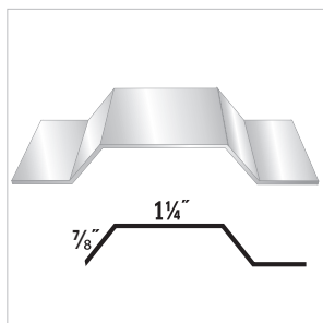
#82 Hat Channel
