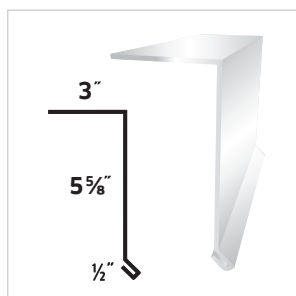
#83 Drip Edge 5 5/8" Face
