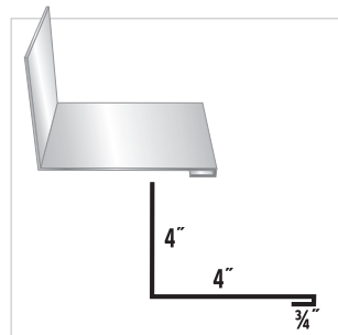
#37 SS Sidewall
