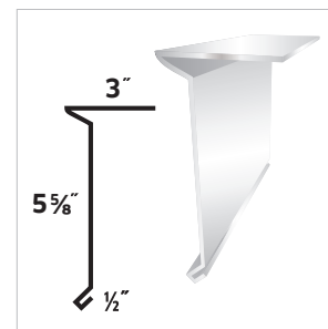
#89 Drip Edge 5 5/8" Extended
