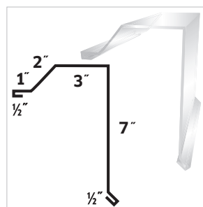
#84 Barn Gable
