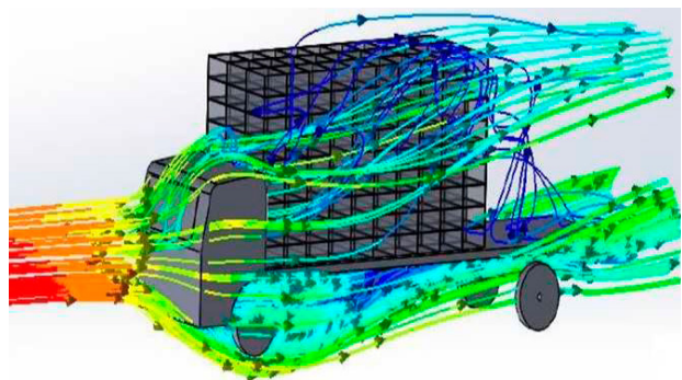
Simulação do movimento do ar durante o transporte de aves (Fonte: PINHEIRO, 2019)
