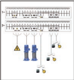
Cuadro eléctrico para GRUPO DE PRESIÓN o RESIDUALES de 2 bombas Protección de nivel de agua y control mediante un contacto (boyas, presostato u otros)
