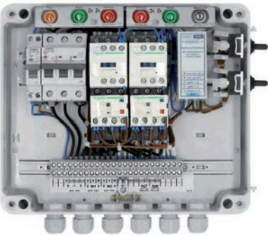
Cuadro eléctrico para GRUPO DE PRESIÓN o RESIDUALES de 2 bombas Protección de nivel de agua y control mediante un contacto (boyas, presostato u otros)
