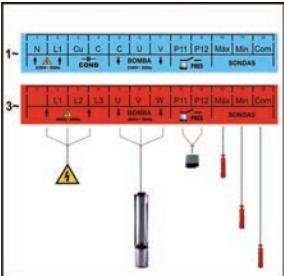
Cuadro eléctrico para BOMBA SUMERGIDA DE POZO de 1 sola bomba Protección de nivel de agua mediante sondas y control mediante un contacto (boya, presostato u otros)
