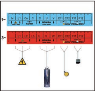
Cuadro eléctrico para GRUPO DE PRESIÓN o RESIDUALES de 1 sola bomba Protección de nivel de agua y control mediante un contacto (boya, presostato u otros)
