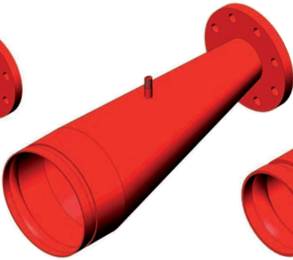
ranura-brida
