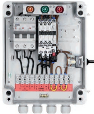
Cuadro eléctrico para GRUPO DE PRESIÓN o RESIDUALES de 1 sola bomba Protección de nivel de agua y control mediante un contacto (boya, presostato u otros)
