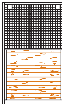
2x8 Tongue & Groove Plank - Mesh Top
