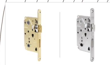
CENTRO foro Wc CENTRO Wc hole
