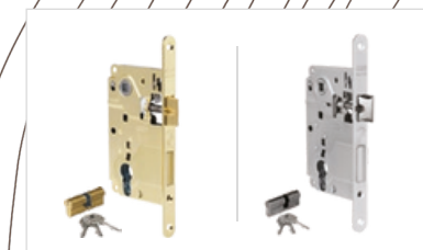
CENTRO Yale + cilindro e 3 chiavi CENTRO Yale + cylinder with 3 keys
