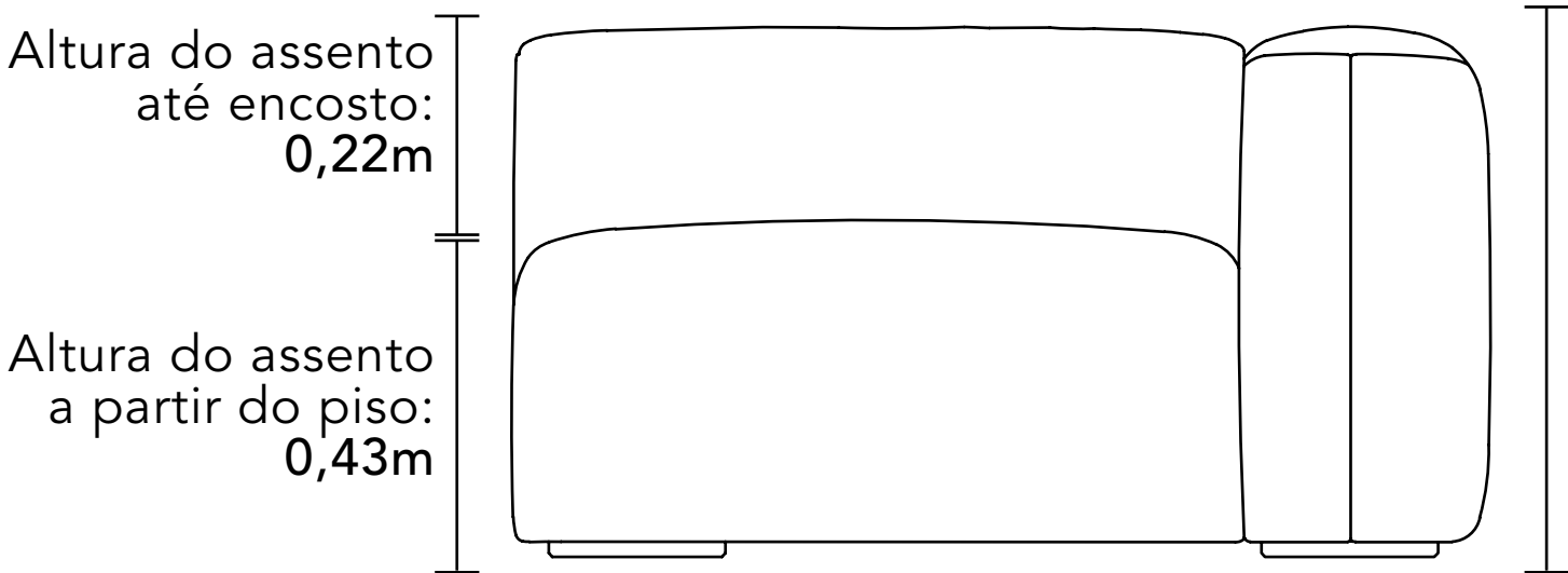
Altura do módulo com encosto: 0,65m
