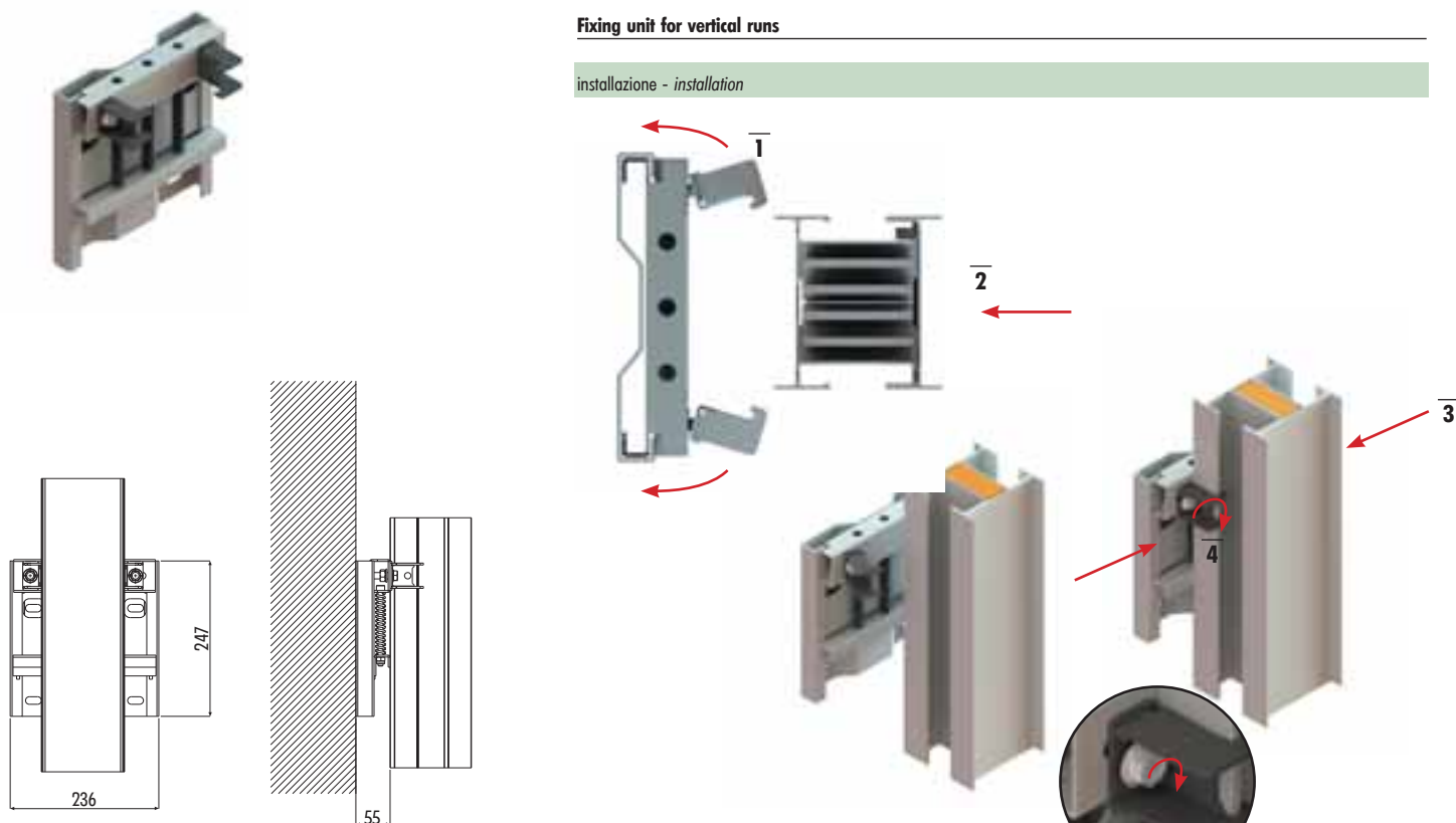
Unità di fissaggio per tratti verticali
