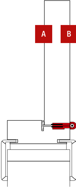
CERNIERE BILICO PIVOT HINGES
