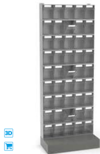
SCAFFALE CON 45 CASSETTI VISUAL BOX DIM. (mm): L=604 P=322 H=1600
