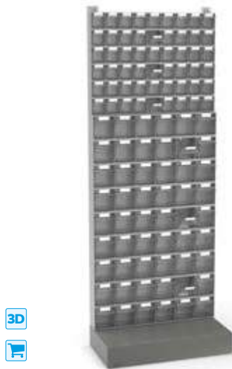
SCAFFALE CON 108 CASSETTI VISUAL BOX DIM. (mm): L=604 P=322 H=1600
