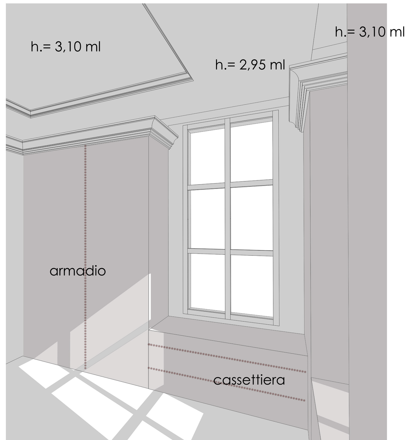
Controsoffitto zona guardaroba vista verso finestra
