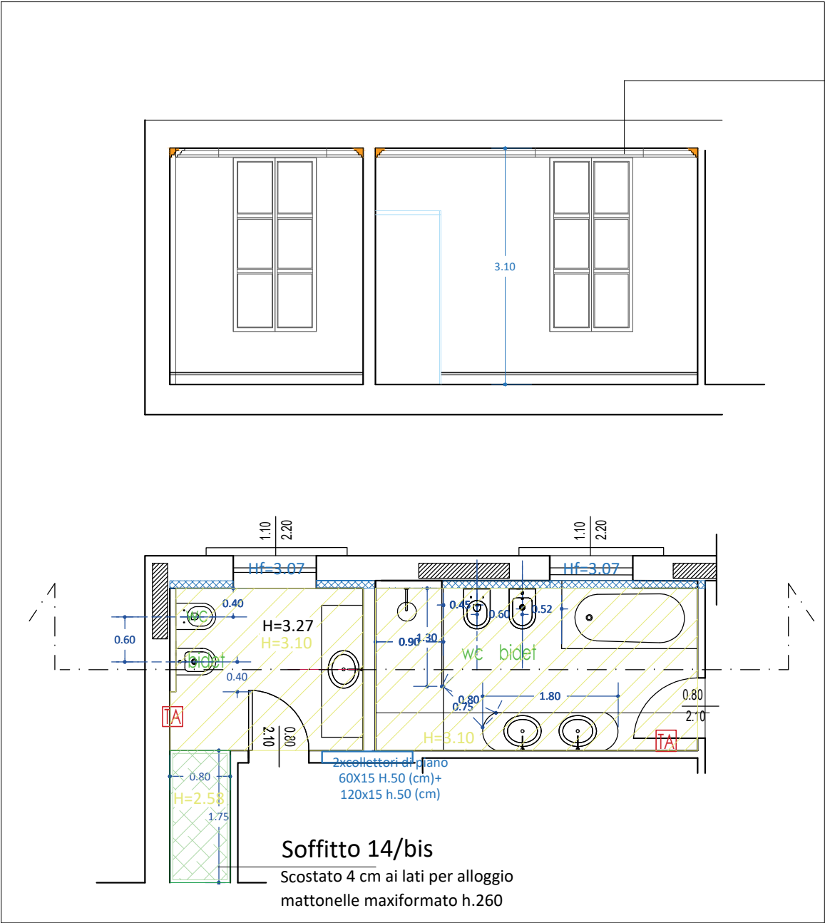
cornice alta max 8/9 cm per evitare intralcio con apertura finestra
