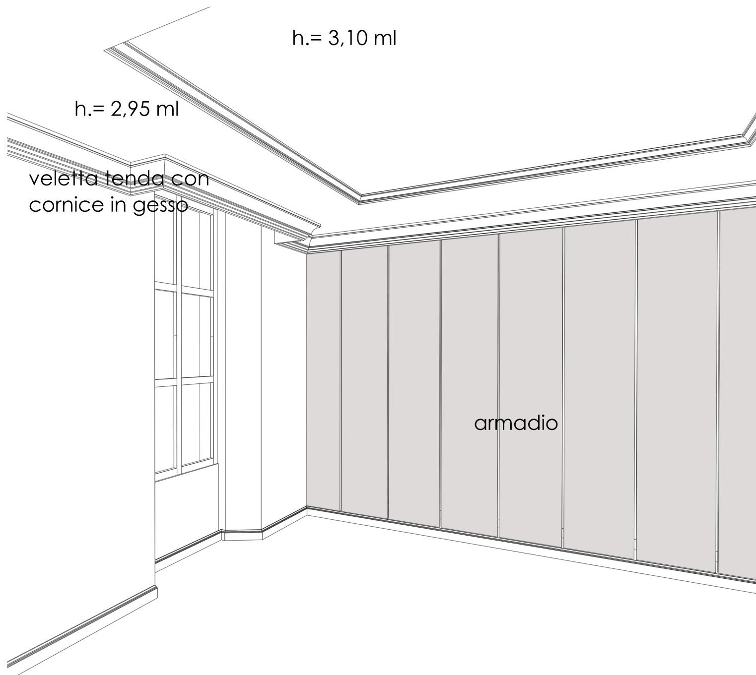
Controsoffitto camera padronale
