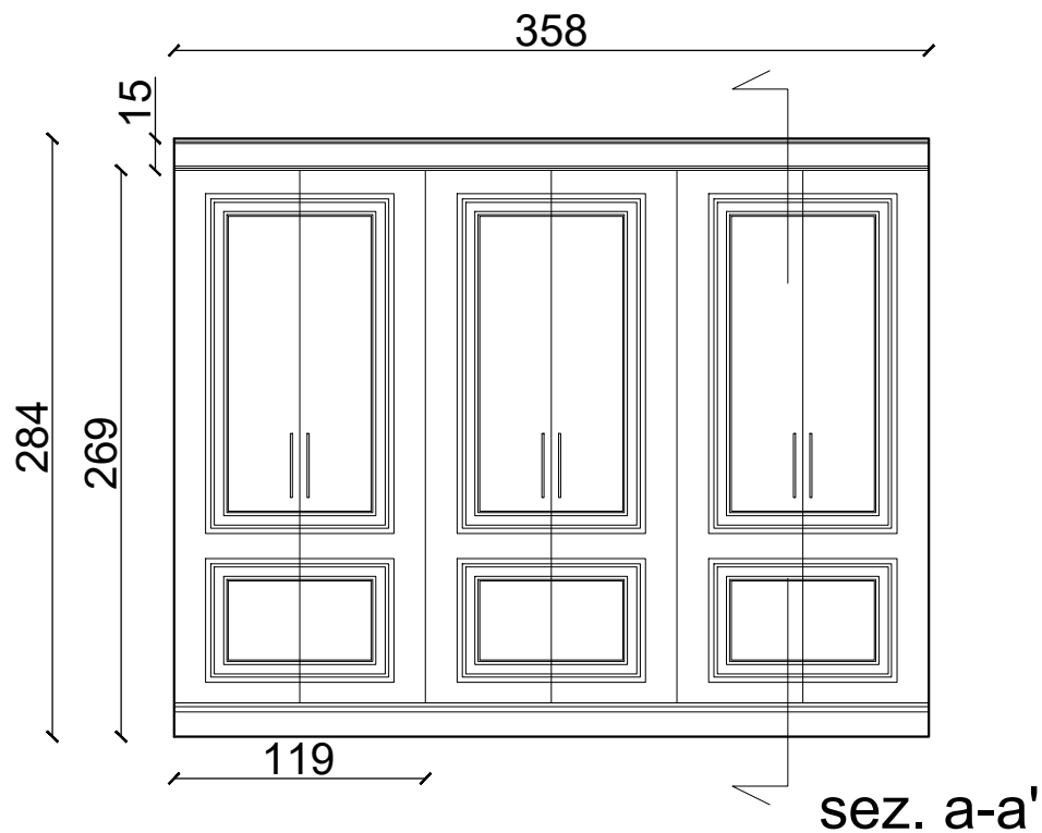
prospetto
