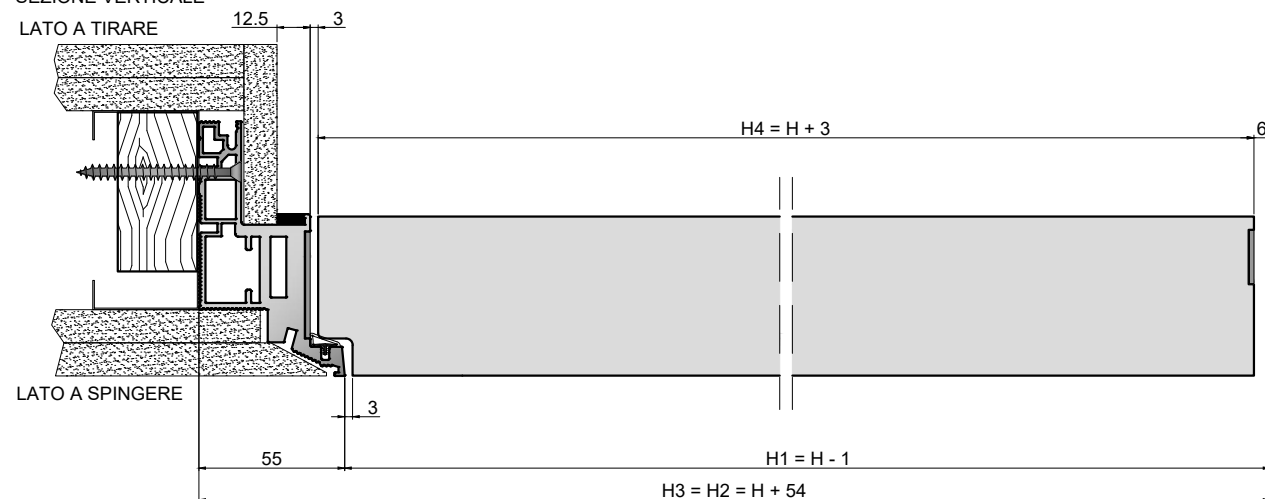
SEZIONE VERTICALE
