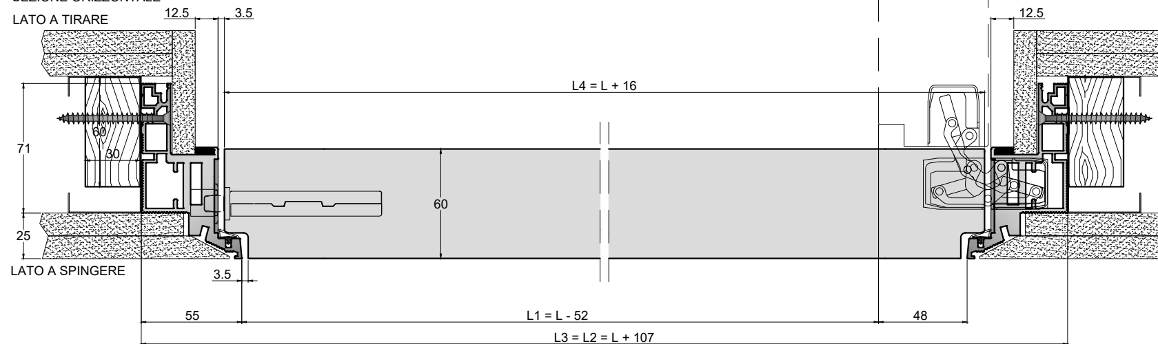
SEZIONE ORIZZONTALE
