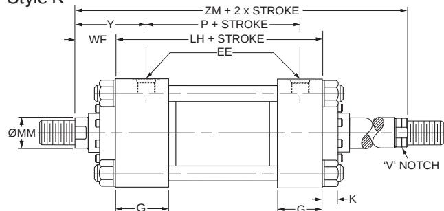
Rod End #1
