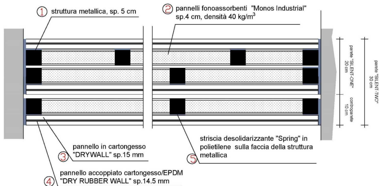
Figura 2_ Stratigrafia della controparete accoppiata alla parete di base: parete "SILENT-TWO" (*)
