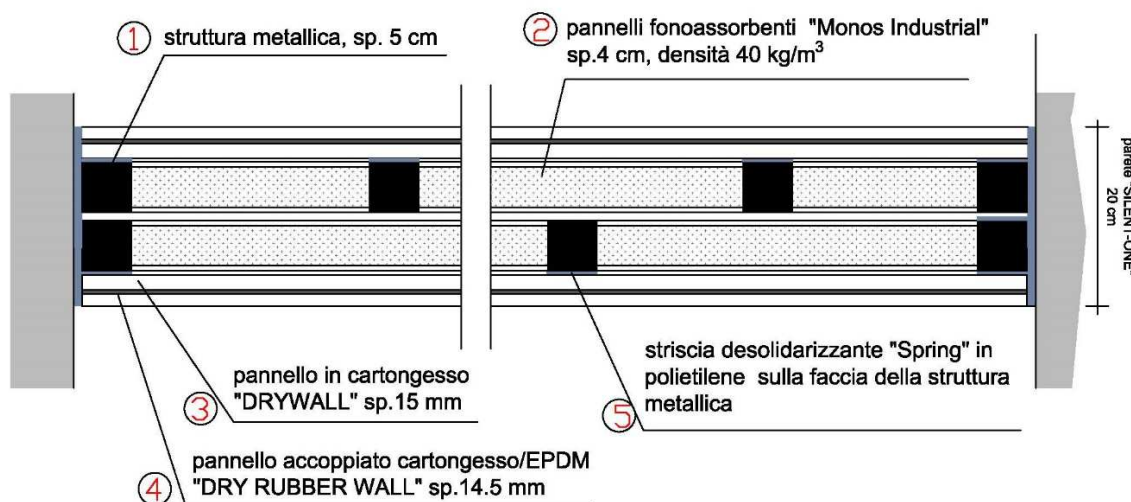
Figura 1_ Stratigrafia della parete di base: parete "SILENT-ONE" (*)
