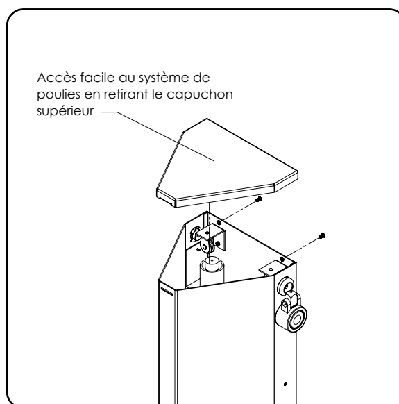
FOCUS SUR LE SYSTÈME DE POULIES
