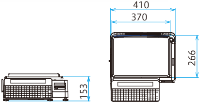
(unit:mm)
