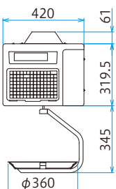
(unit:mm)
