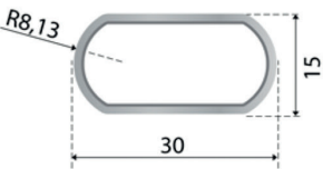
Tubo mecánico elíptico
