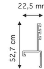
RISCONTRO GUIDA
