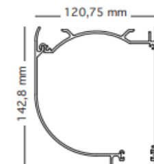
CASSONETTO
