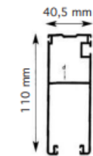
GUIDA IN ALLUMINIO
