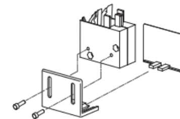
PIEDINO REGOLABILE CON SISTEMA AGGANCIO E SGANCIO
