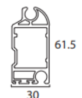
TERMINALE
