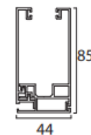
GUIDA
