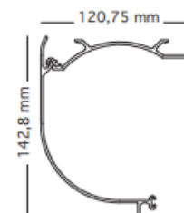
CASSONETTO
