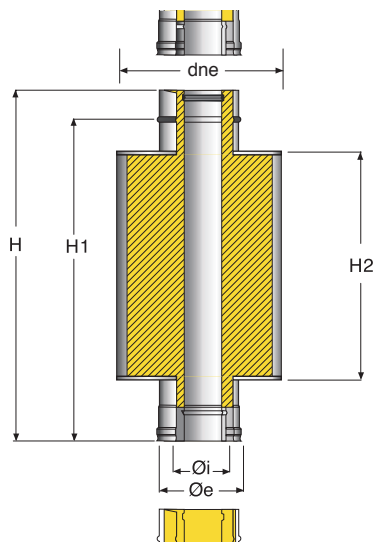
Tubo omologato Gzero per passaggio a tetto - h 1000 mm.
