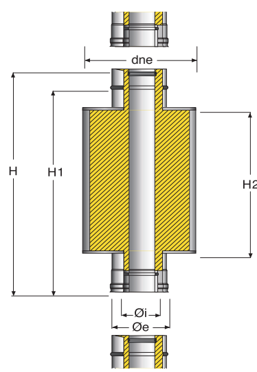
Tubo omologato Gzero per passaggio a tetto - h 700 mm.
