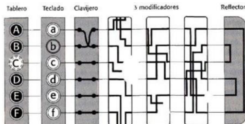
Figura 24. Podemos observar como la adición del clavijero altera el orden de "a" y "b" al intercambiarlas. En la Enigma real habría posibilidad de intercambiar 6 pares de letras.
