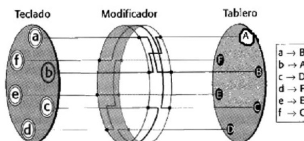
Figura 21 16 . Una versión simplificada de la máquina Enigma con un alfabeto de únicamente 6 letras.
