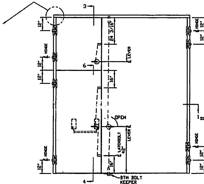
ELEVATION A
