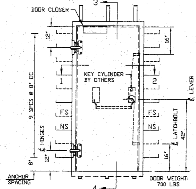
ELEVATION A
