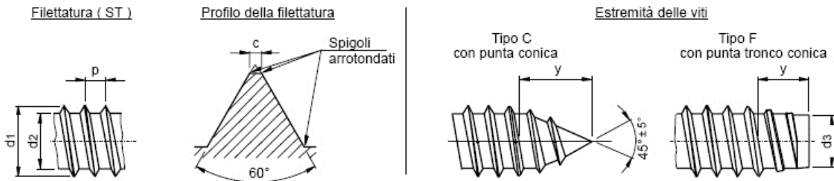
Dimensioni delle filettature dimensioni in mm
