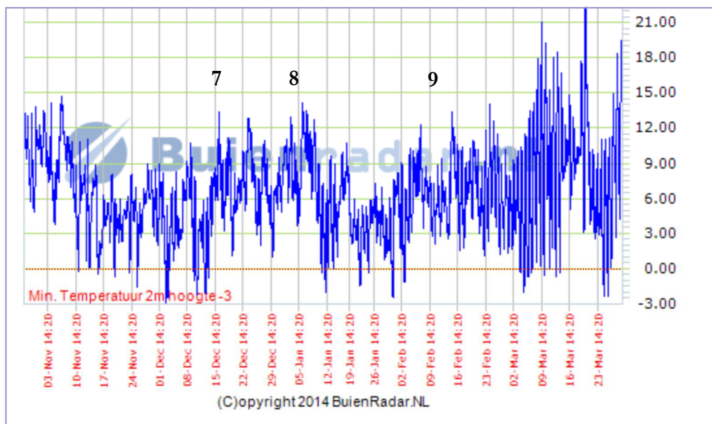
Figuur 2: Temperatuurverloop zoals gemeten door het weerstation ‘Ell’, winter 2013-2014.
