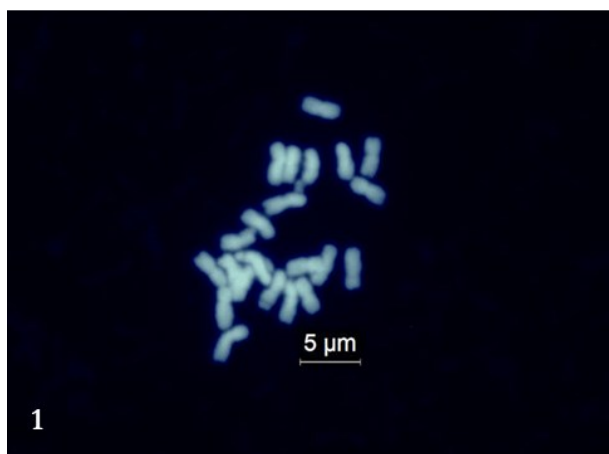
22 chromosomen van F. fulgens 'Gesneriana'
