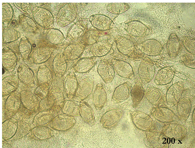
Stuifmeelkorrels van F. triphylla 'PB7760#7'
