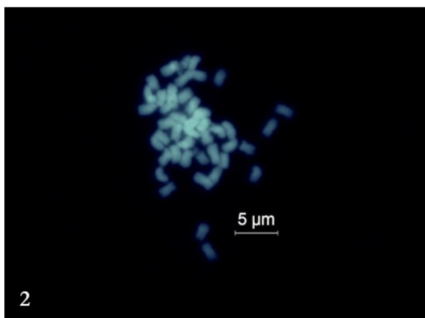
44 chromosomen van F. triphylla 'PB7760#7'
