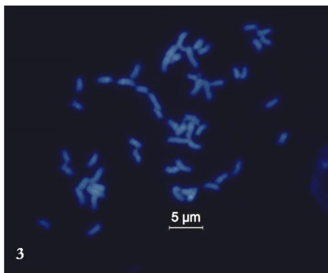
55 chromosomen van 'Göttingen'
