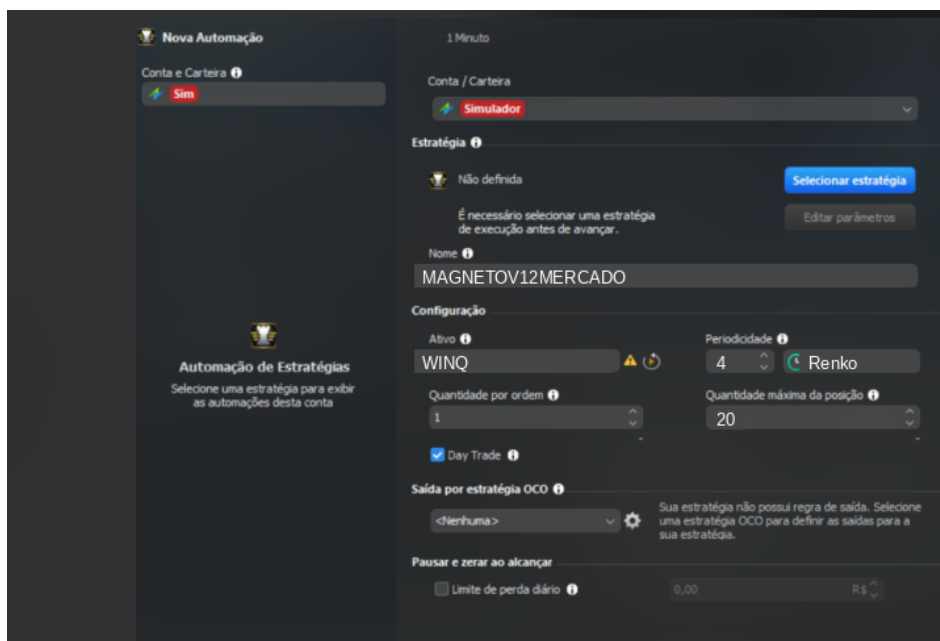
Janela “Nova Automação” com o nome e os parâmetros finais preenchidos.
