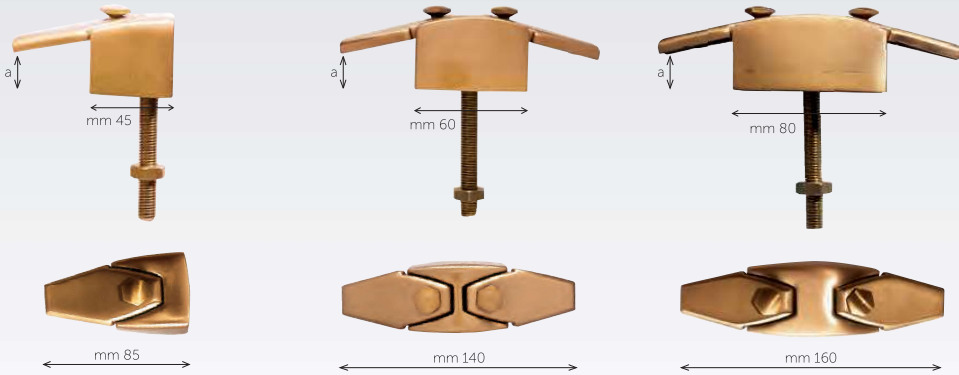
ART. 30770 - a = cm 2-3 Perno da Ø 10 MA x 100 compreso nel prezzo ART. 30773 - a = cm 2-3 Perno da Ø 8 MA x 100 compreso nel prezzo
