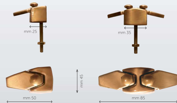
ART. 30977 Perno da Ø 8 MA x 100 compreso nel prezzo
