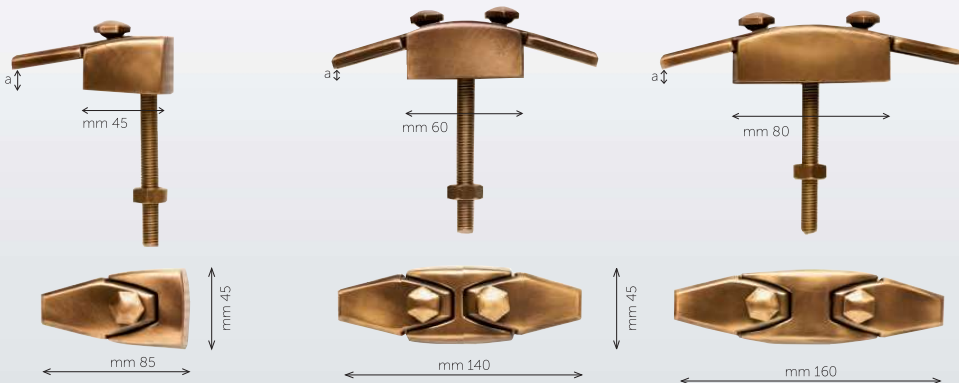
ART. 30930 - a = cm 1-2 Perno da Ø 10 MA x 100 compreso nel prezzo ART. 30942 - a = cm 1-2 Perno da Ø 8 MA x 100 compreso nel prezzo
