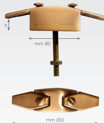
30772 - a = cm 2-3 Perno da Ø 10 MA x 100 compreso nel prezzo 30775 - a = cm 2-3 Perno da Ø 8 MA x 100 compreso nel prezzo
