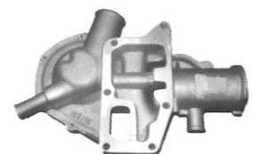
Carcaça da Bomba d'Água Gol CHT com uso de válvula N° Original: 029.121.013-1
