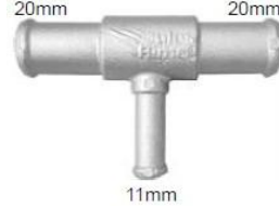
Conexão Mangueira Fiat 2 Saídas Grandes e 1 Saída Pequena
