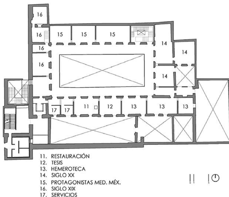
Plano del equipo del proyecto ejecutivo y de la dirección arquitectónica. Planta alta del patio de cárceles restaurada.
