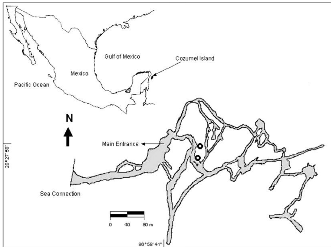
Figura 1. Mapa de localización de la cueva Aerolito de Paraíso, isla de Cozumel, México.
