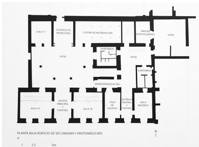
Plano del equipo del proyecto ejecutivo y de la dirección arquitectónica. Planta baja de la Secundaria y el Protomedicato restaurada.
