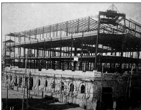
El arquitecto fue el italiano Adamo Boari y los cálculos y concepción estructural, estuvieron a cargo de don Gonzalo Garita. Foto: https://i.pinimg.com/originals/80/cb/d6/80cbd69fa6b26418581fcbcc42d6c2e0.jpg
