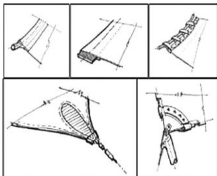
Tipos de relingas. [Fuente: http://wiki.ead.pucv.cl/index.php/Tensado_Estructural ]
