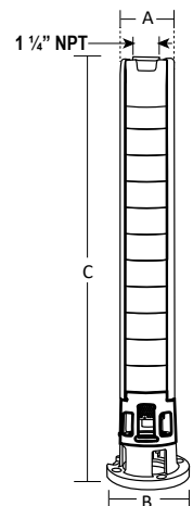
Acoplamiento NEMA 6"
