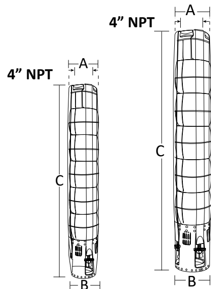
Acoplamiento NEMA 6"
