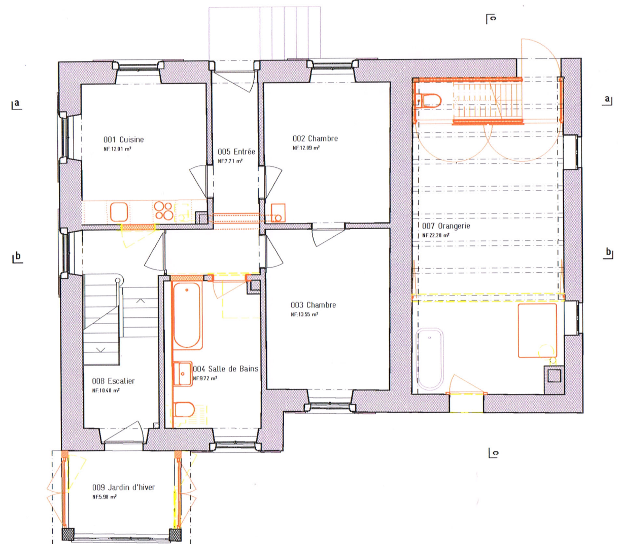
Premier étage
