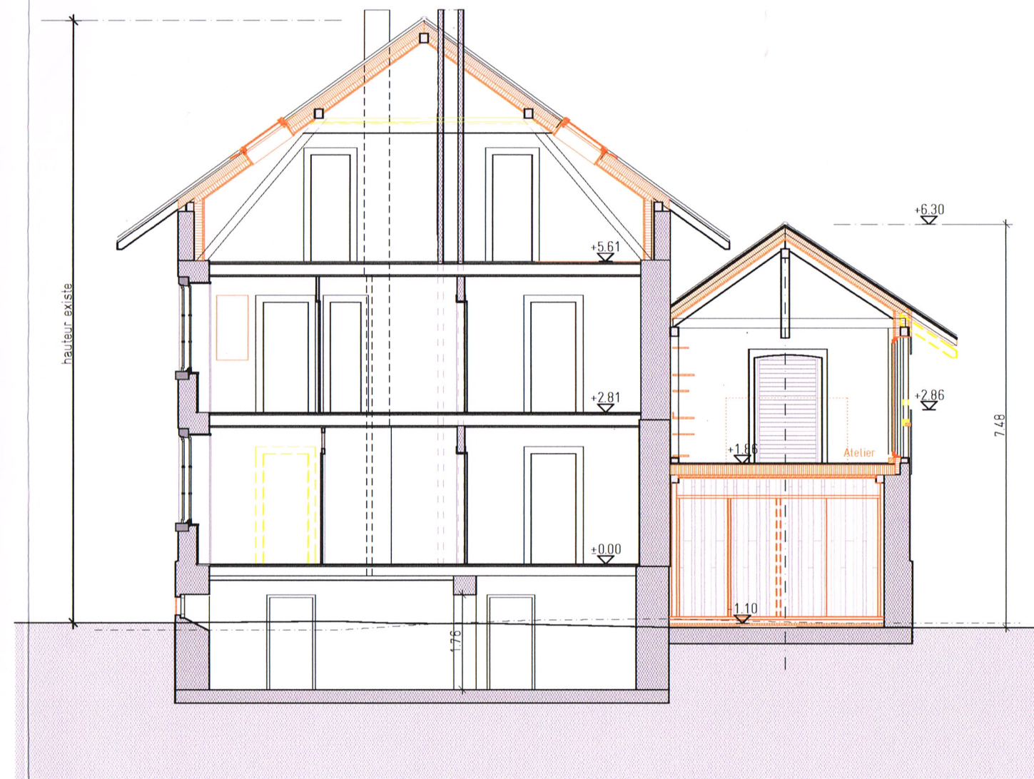
Coupe c-c
