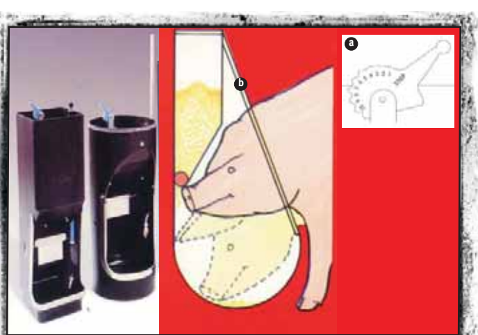
f Foto 5.10. Comedero tolva con dosificador. a) mecanismo dosificador; b) funcionamiento de la compuerta.
