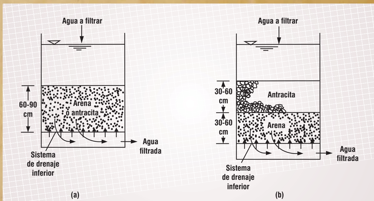
Figura 12.2. Tipos de filtros empleados para la filtración del agua residual. (a) Filtro convencional, monomedio, flujo descendente (b) Filtro convencional bimedio, flujo descendente
