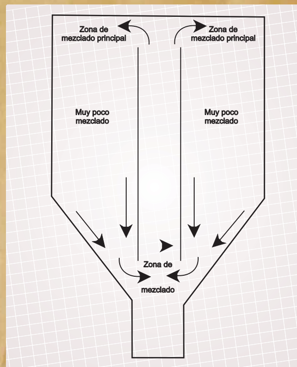
Figura 5.6. Flujo típico del alimento en un mezcladora vertical.
