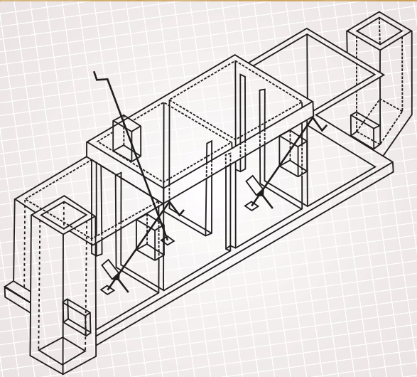
F Figura 12.5. : Esquema de reactor vertical.
