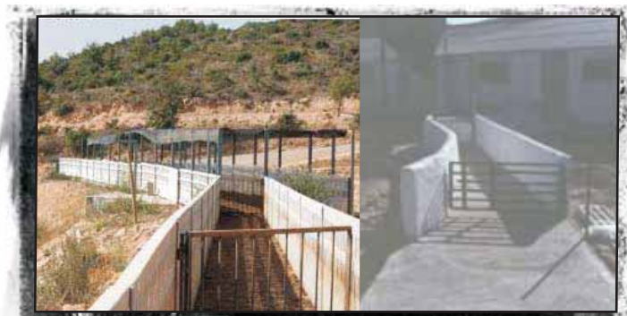
f Foto 13.2. Los pasillos deben tener la menor cantidad de giros posibles.
