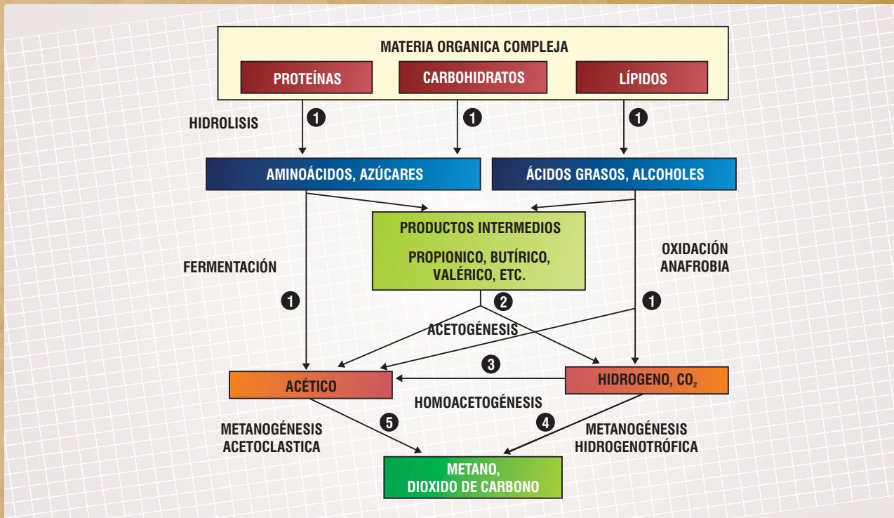
Figura 12.3. Esquema de reacciones de la digestión anaerobia de materiales poliméricos.
