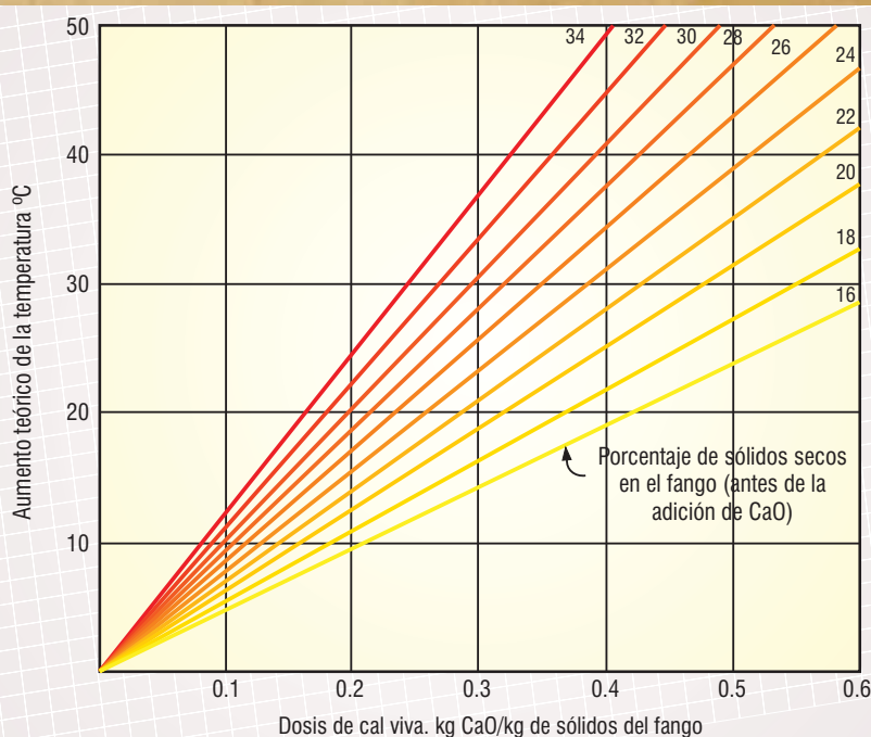
Figura 12.7. Aumento teórico de temperatura en fangos post-estabilización con cal viva.
