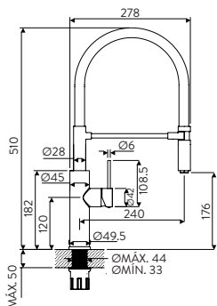
HOOP 20-202N / 20-202NI
