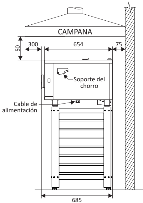
Lado Derecho
