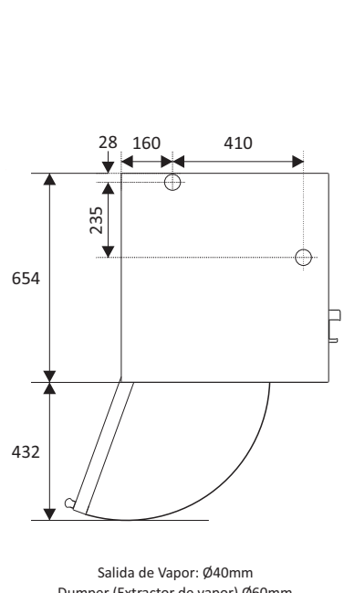
Vista Superior
