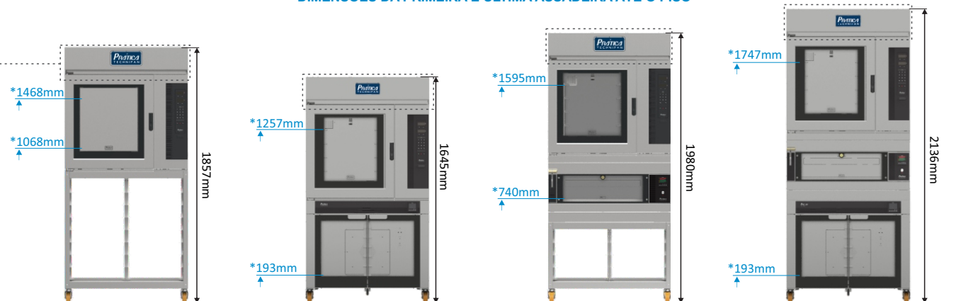
HPE100 PROGRAMÁVEL BASE 16 ASSADEIRAS
