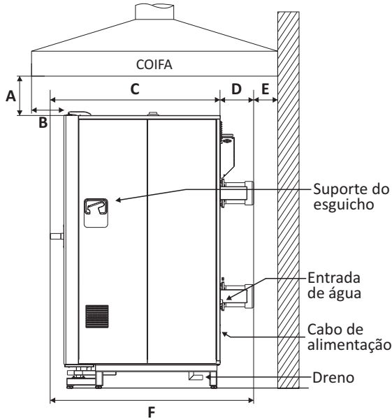
VISTA LATERAL
