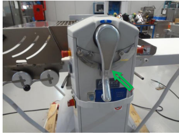
Alavanca de regulagem e escala de graduação para ajuste de espessura
