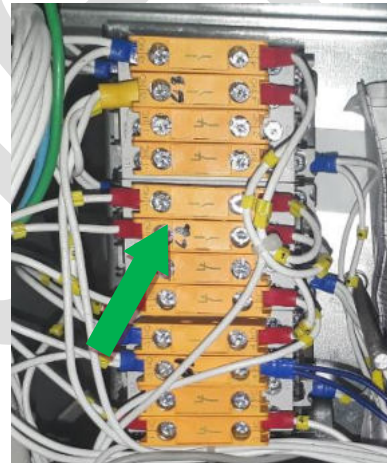
Contator com contatos positivamente guiado
