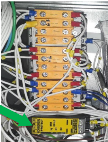
Relé de Segurança da Marca Schmersal SRB 201LC categoria 4
