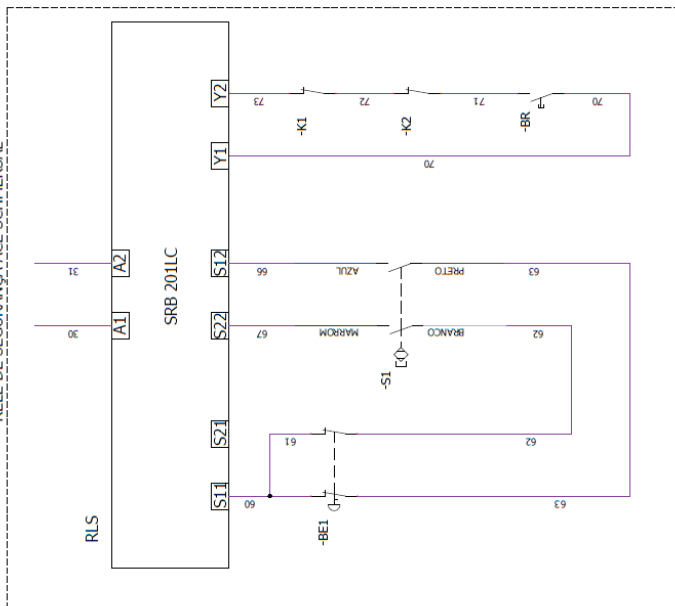
RELÉ DE SEGURANÇA ACE SCHMERSAL
