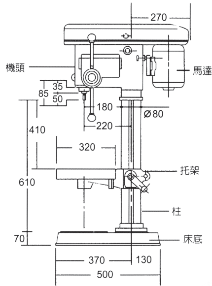
◀TD-120 TD-14 TDT-340 機械各部名稱及尺寸
