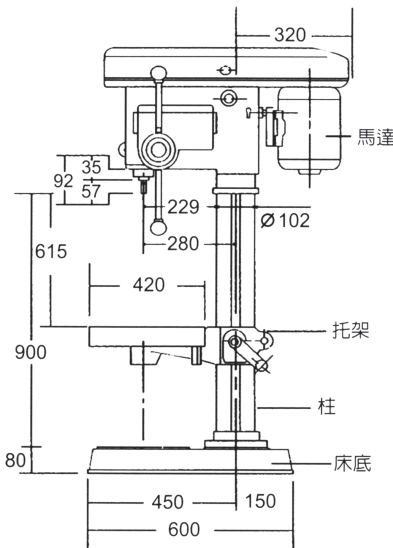
◀TD-250 TD-25 TDT-25 TDT-32 機械各部名稱及尺寸
