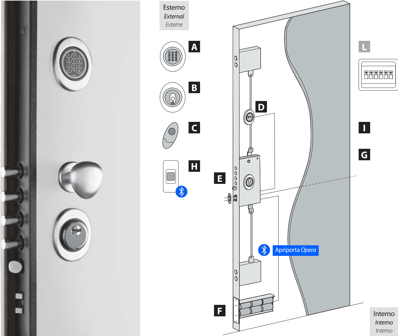
Vista esterna con tastiera External view with keyboard Vue extérieure avec clavier
