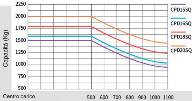
Curva di carico
