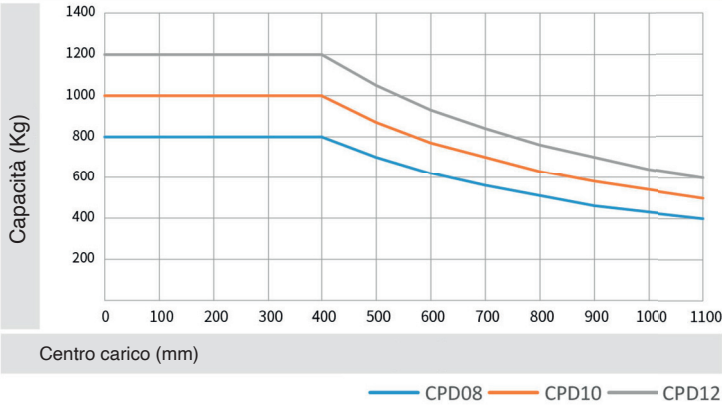
Curva di carico
