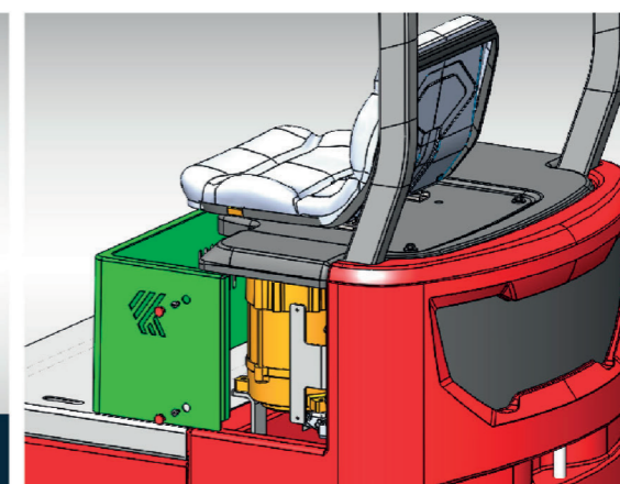
Schema del layout del controllo elettrico
