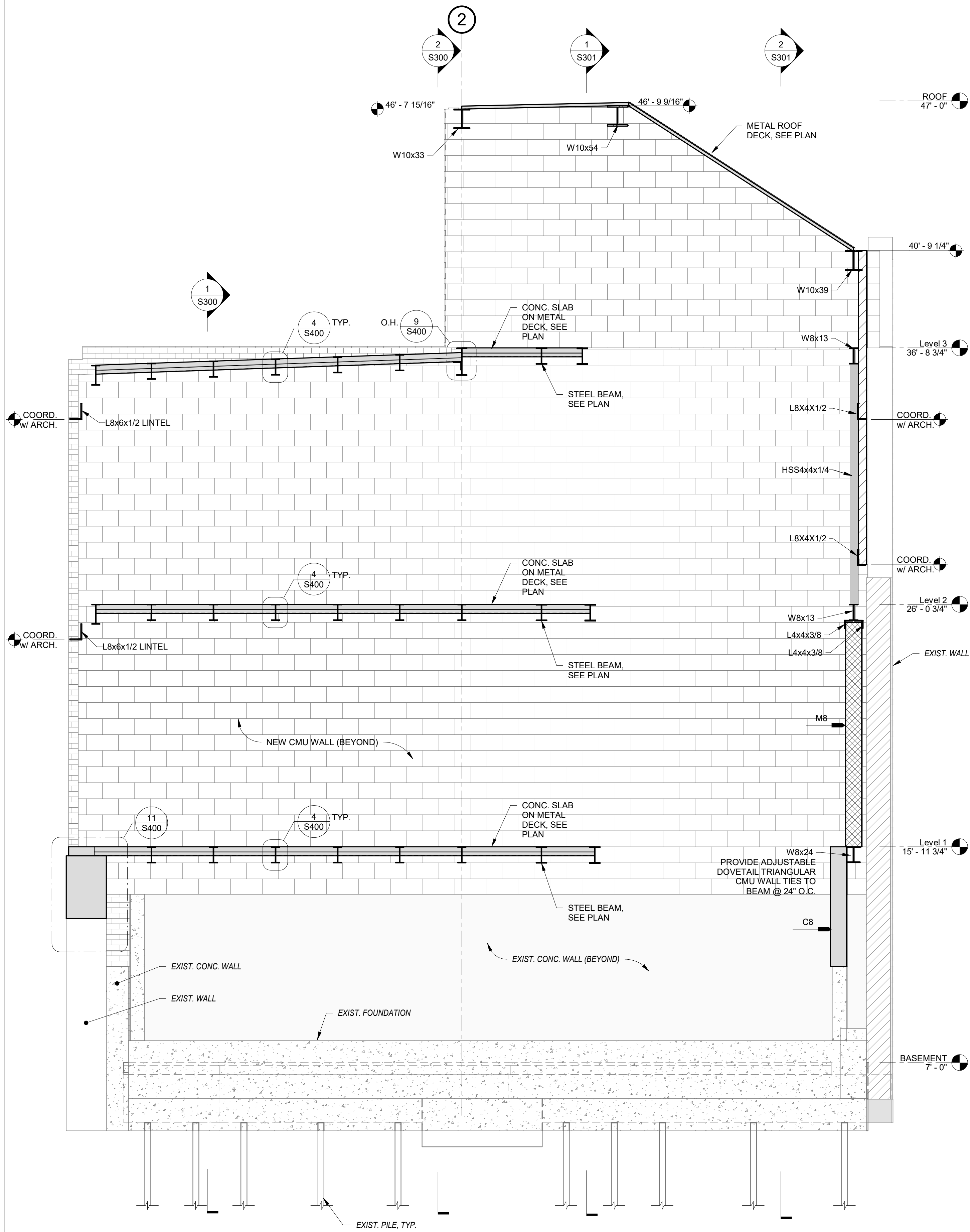
1 SECTION SCALE: 3/8" = 1'-0"
