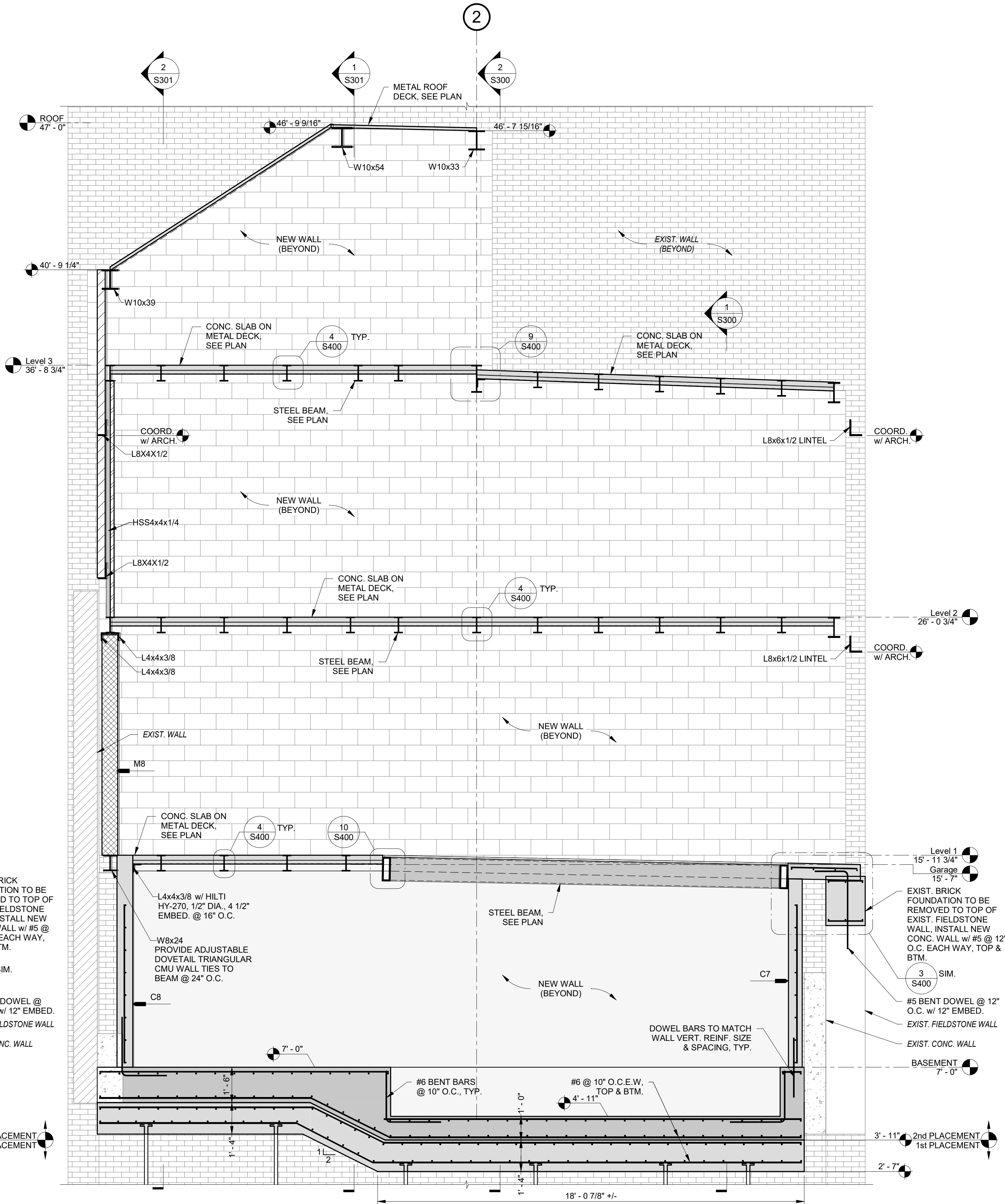
2 SECTION SCALE: 3/8" = 1'-0"
