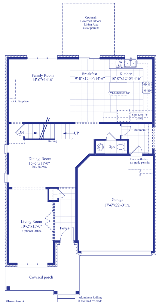
Elevation A
