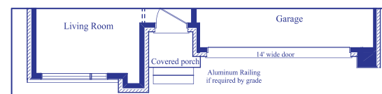
Elevation B
