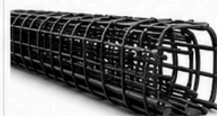
CAGES D'ARMATURES
